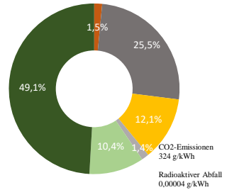
verbleibender Energieträgermix
