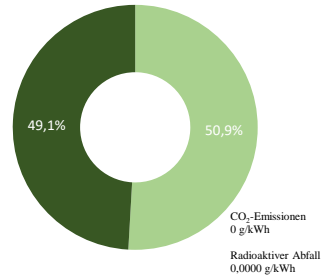
verbleibender Energieträgermix
